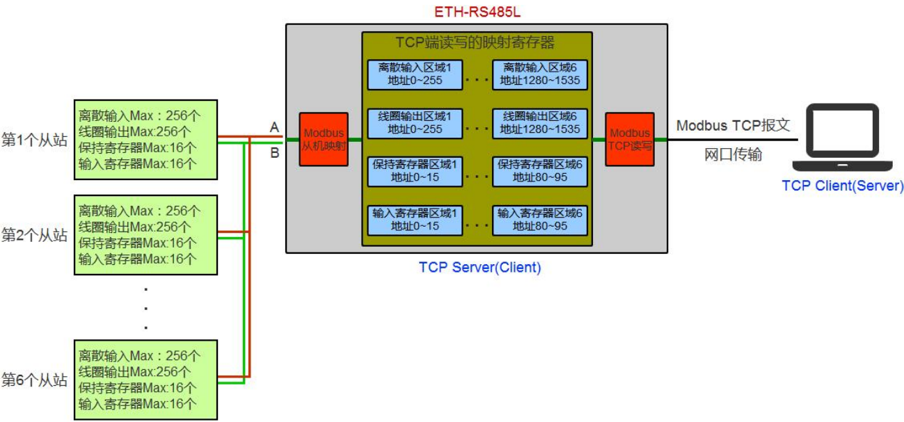
Figura 5.5.1 Diagrama de la función de mapeo de esclavos Modbus
