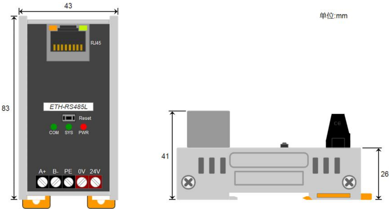
Figura 3.1 Dimensiones de ETH-RS485L
