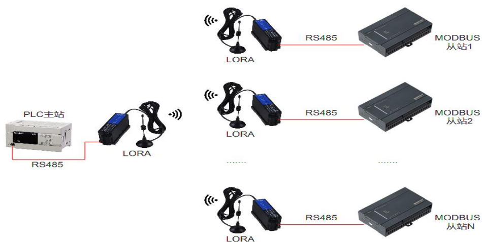
Figura 5.1.2.2 Caso de comunicación punto a muchos
