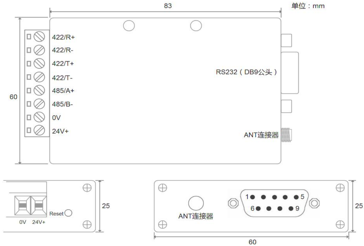
Figura 3.1 Diagrama de dimensiones RS232/485/422-LORA
