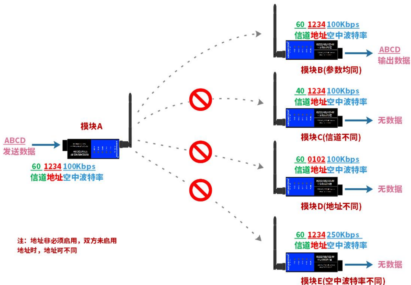
Figura 5.1.1 Transmisión punto a punto
