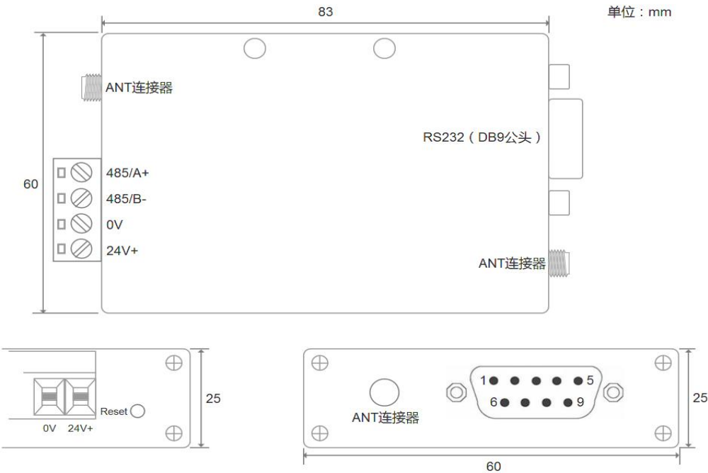
Figura 3.1 Diagrama de dimensiones de RS232/485-LORA-Pro
