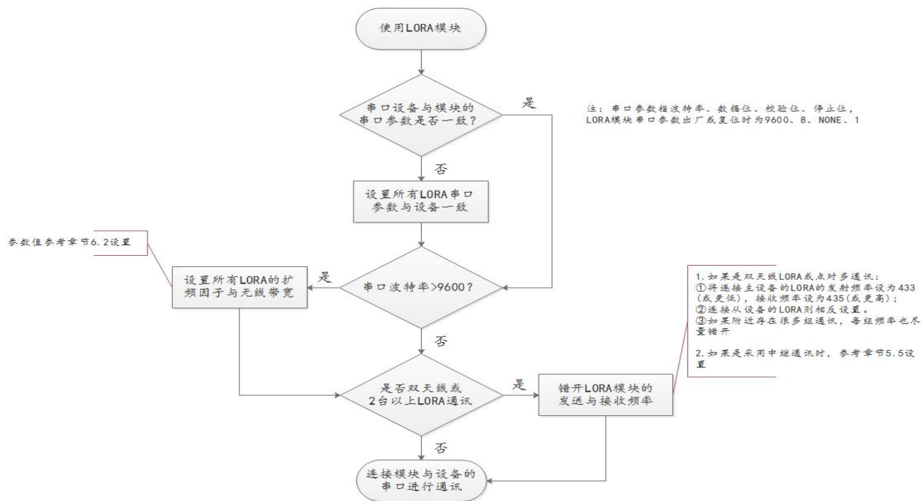
Figura 4.1 Flujo de uso general del módulo LoRa
