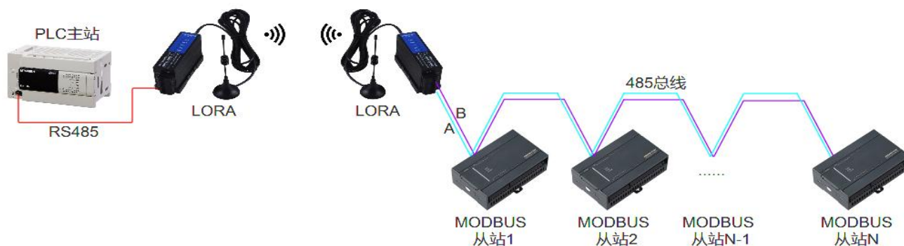
Figura 5.1.1.3 Comunicación multidispositivo punto a punto
