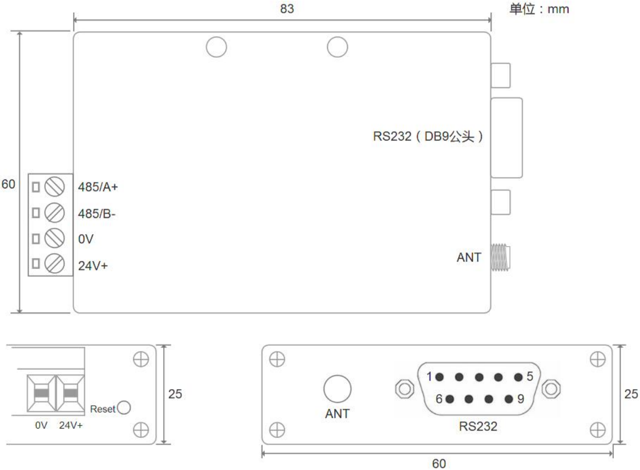
Figura 3.1 Dimensiones de RS232/485-LORA-T
