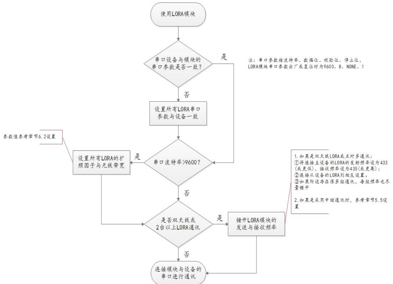
Figura 4.1 Flujo de uso general del módulo LoRa
