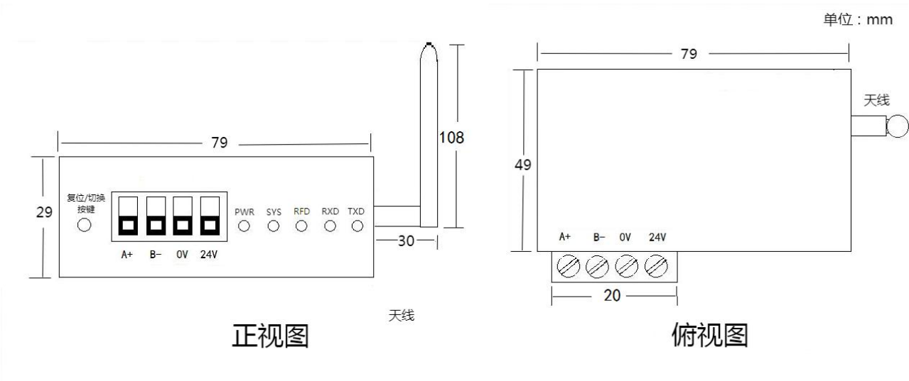
Figura 2.2 Dimensiones de RS232-WIFI-M01
